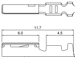
リセプタクルコンタクト
