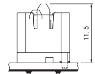
PHN连接器接插时 (带标准定位柱)
