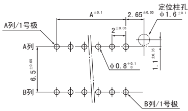
(带标准定位柱)
