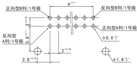
(带标准定位柱)
