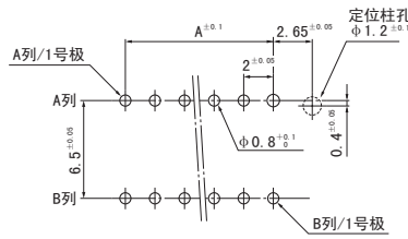
(带小型定位柱)
