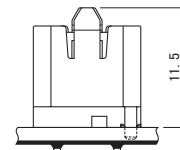
KR连接器接插时 (带标准定位柱)
