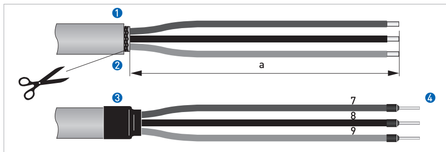
Figure 12: Cabo de corrente de campo, preparação para sensor de medição
