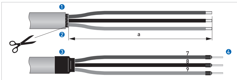
Figure 9: Cabo C de corrente de campo, preparação para o conversor de sinal
