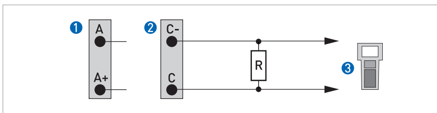
Figure 43: Ligação HART® activa (I a )
