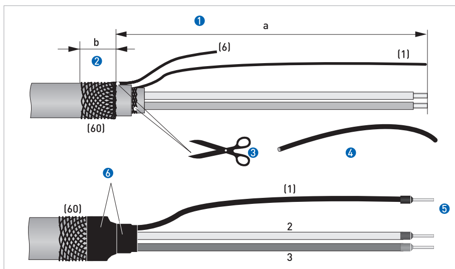
Figure 10: Prepare o sinal de cabo A, ligue ao sensor de medição
