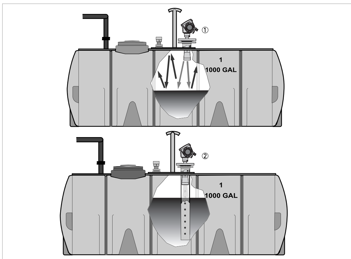
Obrázek 3-11: Vodorovná válcová nádrž
