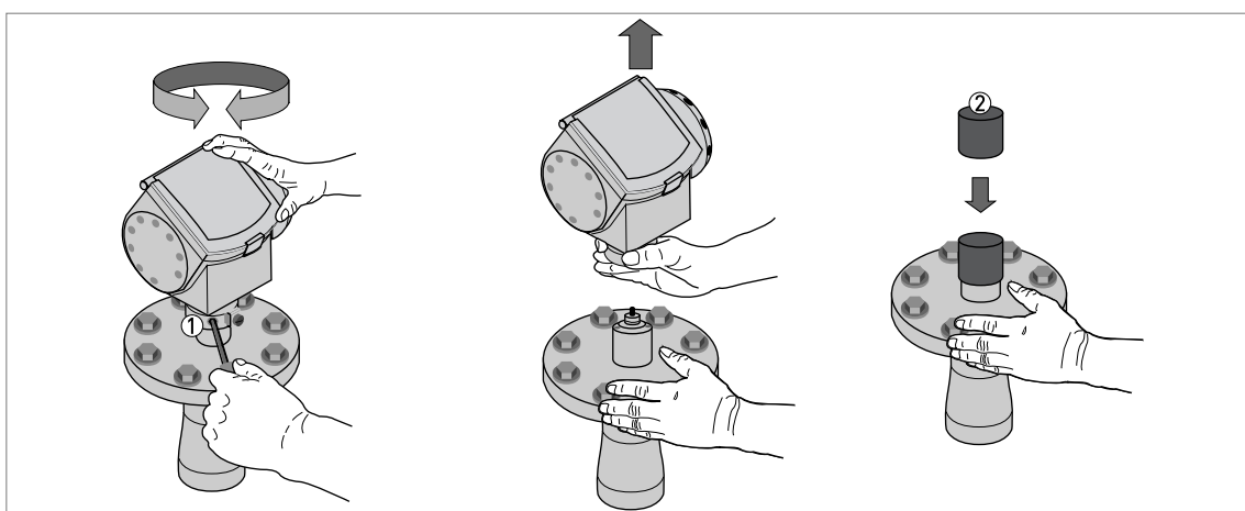
Obrázek 3-24: Jak natočit nebo demontovat převodník signálu
