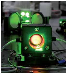
Ultrafast lasers
