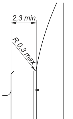
Einzelheit X detail X
