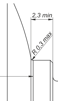
Einzelheit Y detail Y
