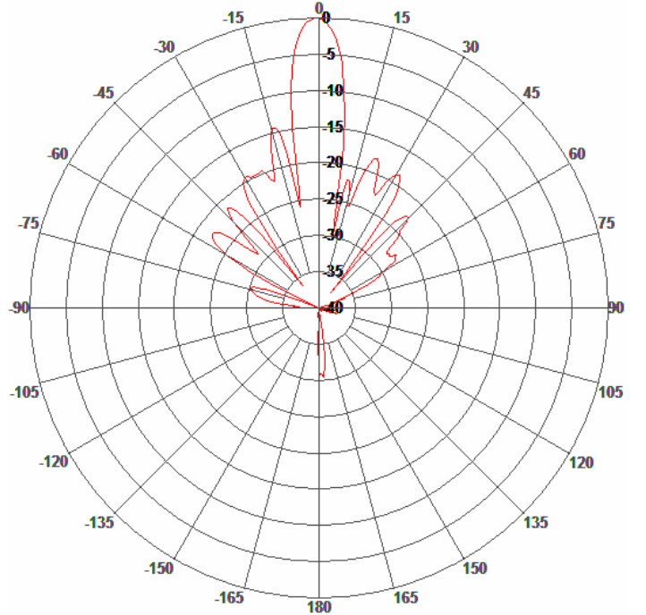
H-Plane Pattern
