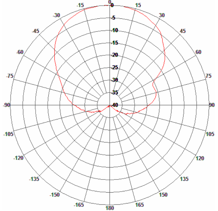
H-Plane Pattern
