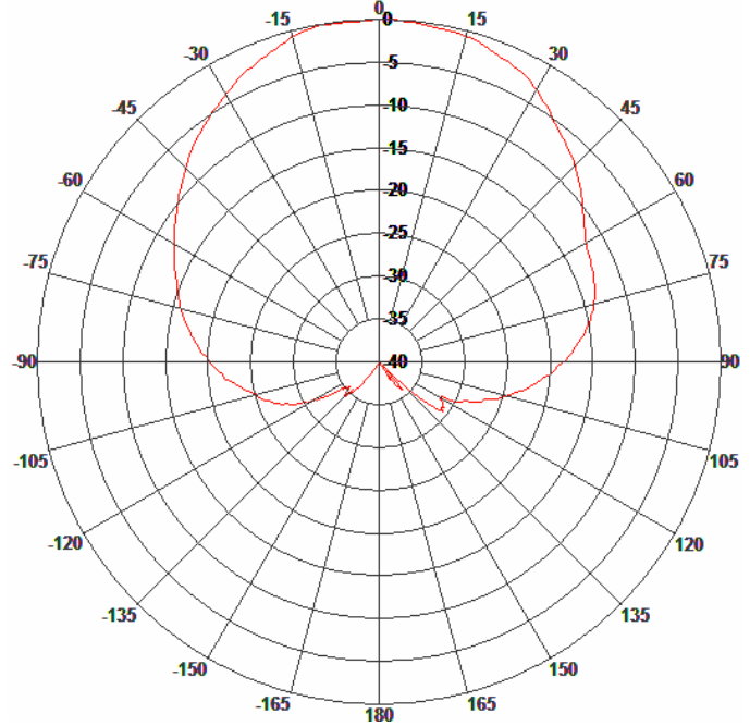
H-Plane Pattern
