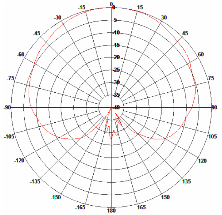
H-Plane Pattern
