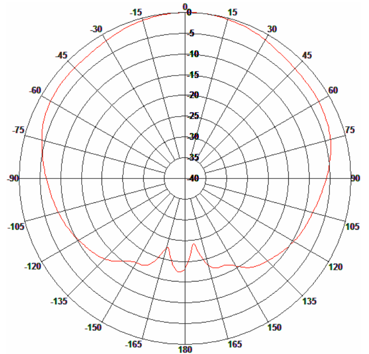
H-Plane Pattern
