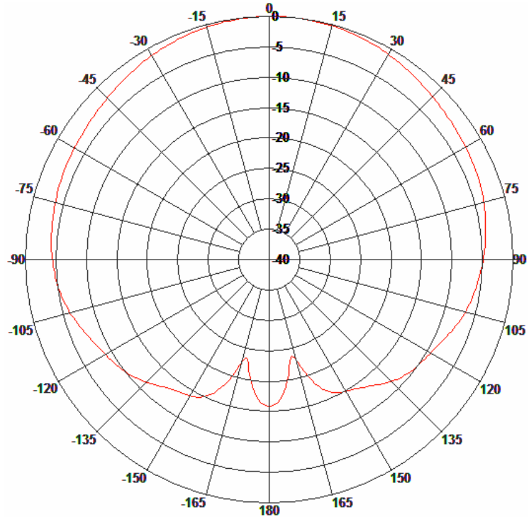
H-Plane Pattern
