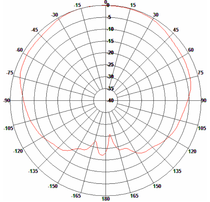
H-Plane Pattern
