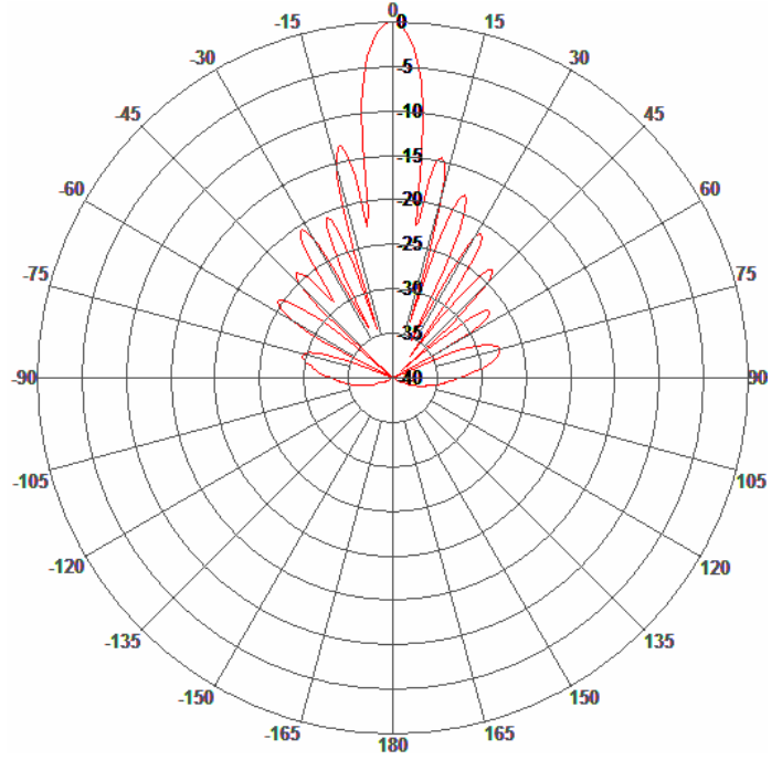
H-Plane Pattern
