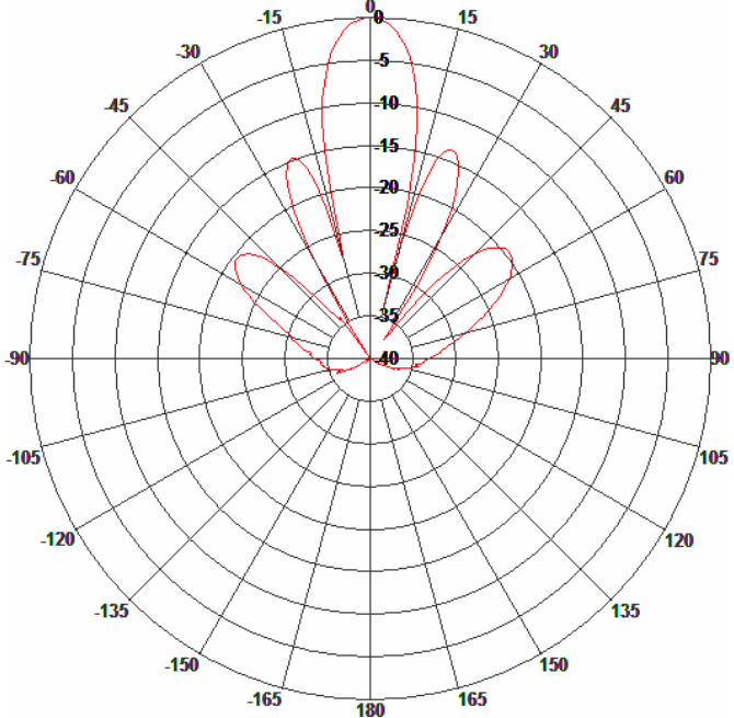
H-Plane Pattern
