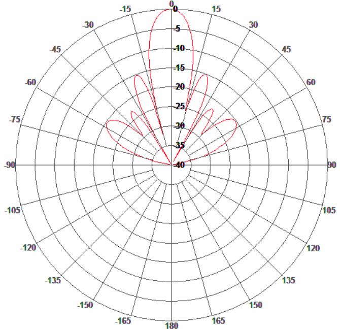
H-Plane Pattern
