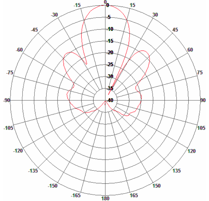
H-Plane Pattern
