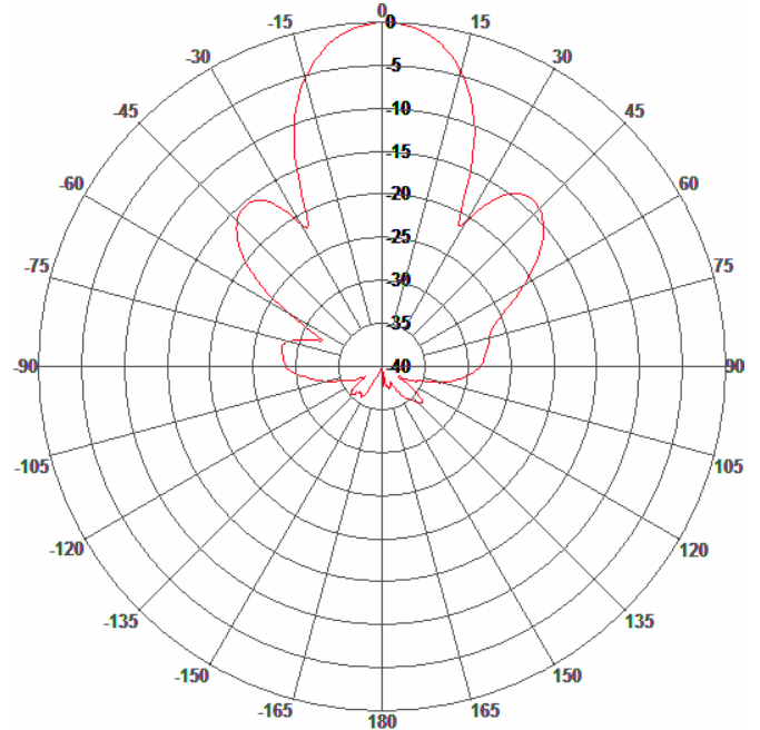
H-Plane Pattern
