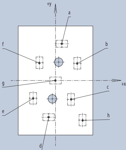
Montagebohrung
