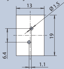
Montagebohrung
