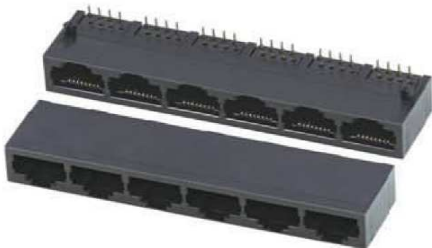
P4113-00GXX1 5921-1X6-8C(4C)
