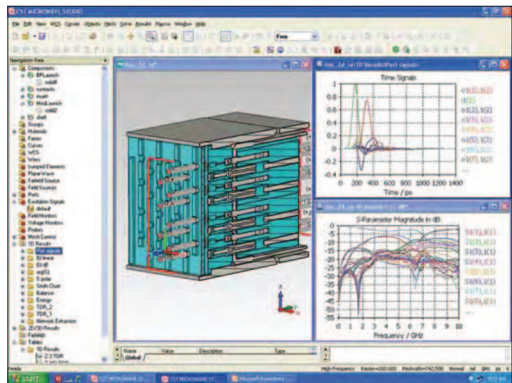
3DEM Model/S-Parameter
