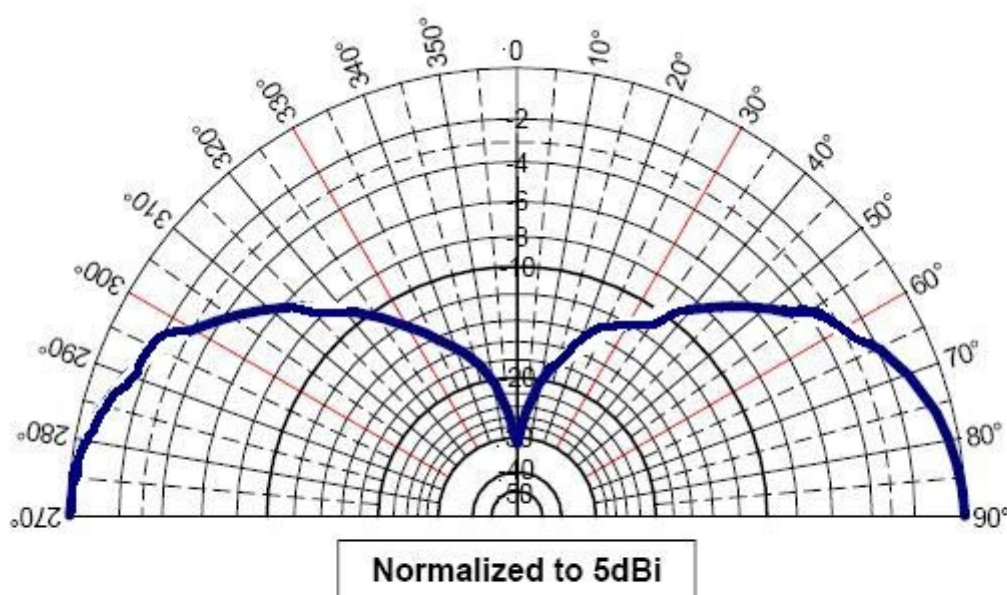
Elevation Pattern (Z, Y or H-Plane)
