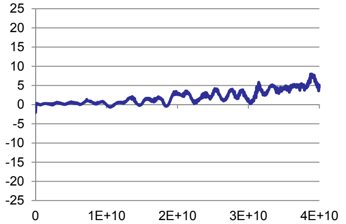
Phase Balance S31-S41
