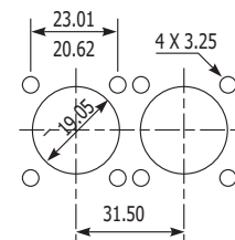
Viereckiger, fest angebrachter Steckverbinder, Montage von hintenvon hinten
