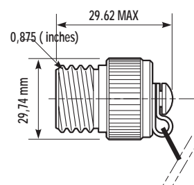
Schutzstöpsel für Viereckiger, fest angebrachter Steckverbinder (Nylonschnur)
