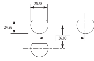
Plattenschneider - runder, fest angebrachter Steckverbinder, Montage von hinten
