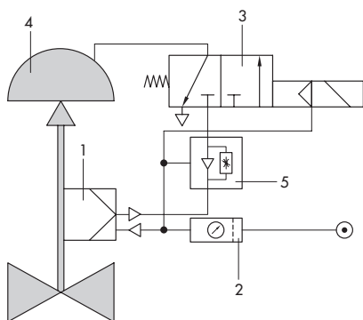
Obr. 6: Instalace zesilovače objemového průtoku s přidavným magnetickým ventilem
