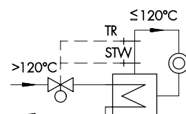
3. ábra - Fűtőberendezés kombinált hőmérséklet-szabályozóval és biztonsági hőmérséklet-törrel a DIN 4751 szerint
