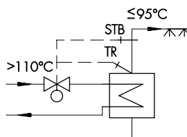
5. ábra - Vízfűtő berendezés hőmérséklet-szabályozóval és biztonsági hőmérséklet-határolóval a DIN 4753 alapján
