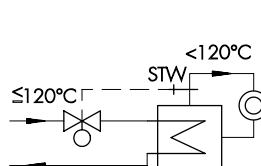
2. ábra - Fűtőberendezés biztonsági hőmérséklet-törrel a DIN 4747 szerint
