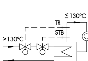
4. ábra - Forróvíz fűtőkészülék hőmérséklet-szabályozóval és biztonsági hőmérséklet-határolóval a DIN 4752 szerint
