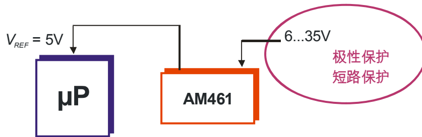
图8: 微处理器供电电路
