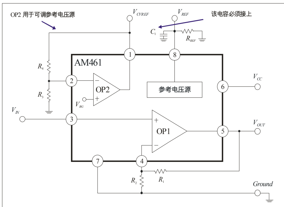
图4: 可调恒压源
