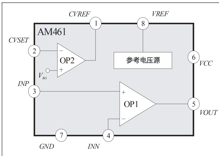
图1: AM461电路方框图
