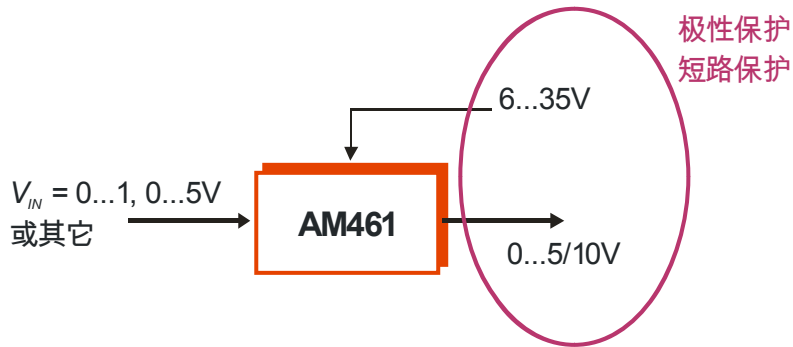
图7: 作为放大和阻抗变换电路
