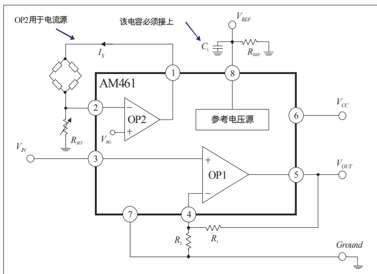
图3：可调恒流源
