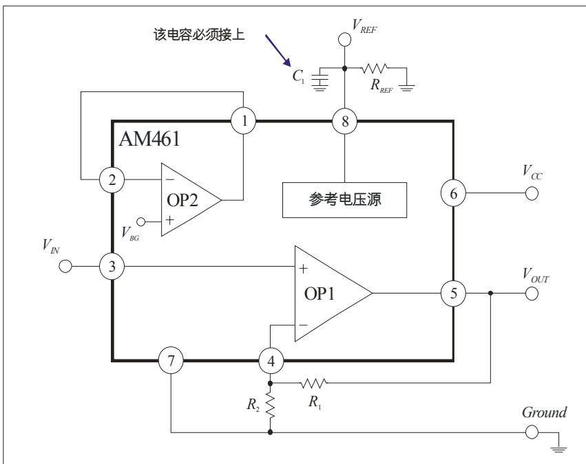
图2：放大器的典型应用
