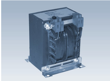
Fußwinkel-Transformator mit Anschlußklemmen
