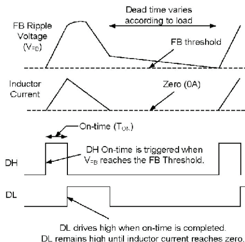
Fig. 28 - Power-Save Mode
