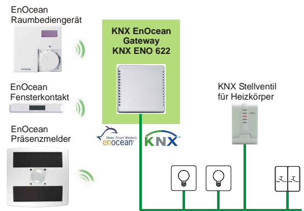
Abb. 6: Anwendungsbeispiel Heizungsregler
