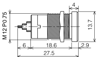
RECEPTACLE
