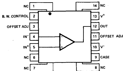
(outline dwg FD)
