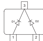
BAT54-05 BAT54-05W
