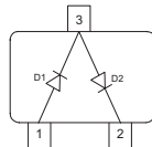
BAT54-04 BAT54-04W
