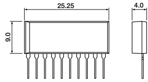
STA 10pin
