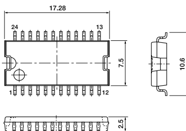
SPF24pin
