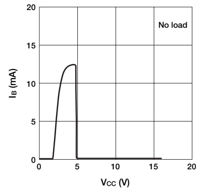
■ V_S Input Current
