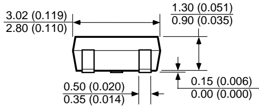
SOT-23-5 (M)
