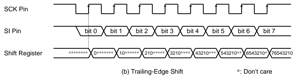
Figure 15.24 Shift Edge Types
