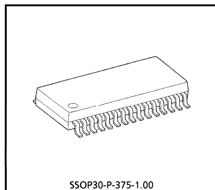
SSOP30-P-375-1.00
