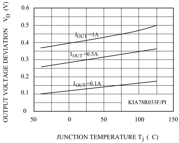
Fig.12 V_D - T_j
