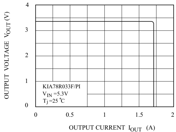
Fig. 11 V_{OUT} - I_{OUT}
