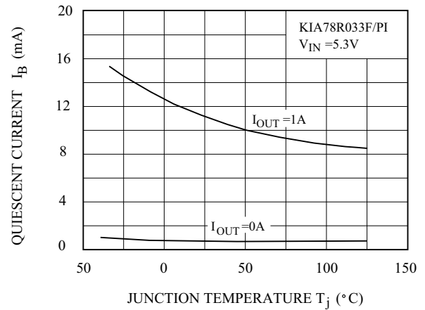
Fig. 9 I_B - T_j
