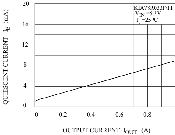
Fig. 10 I_B - I_{OUT}
