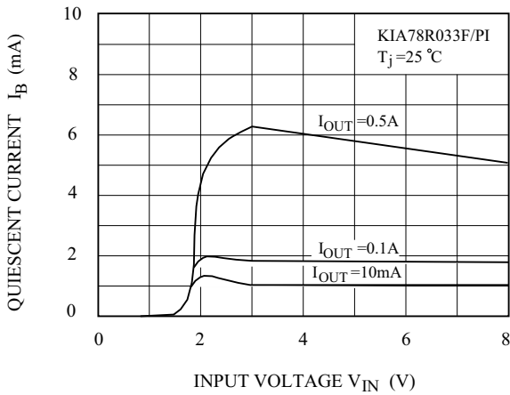
Fig. 8 I_B - V_{IN}
