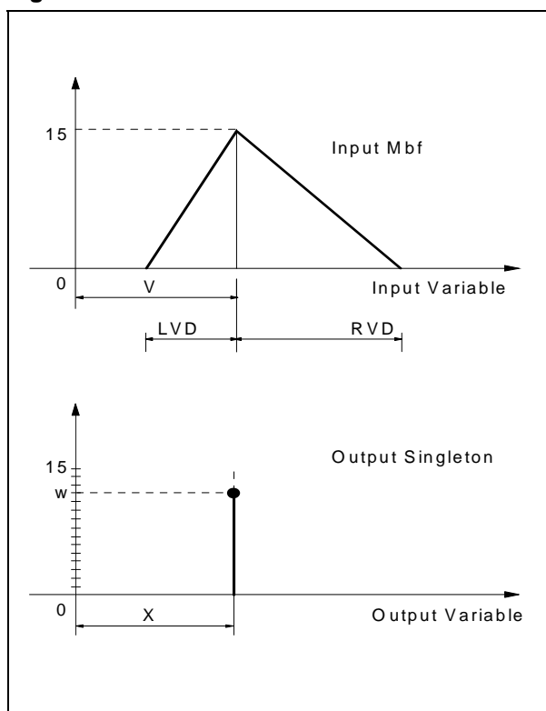
Figure 2.10 Mbfs Parameters
