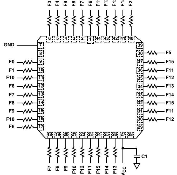
MR82C55A CLCC
