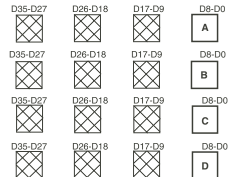
(d) x18 INPUT to x36 OUTPUT
