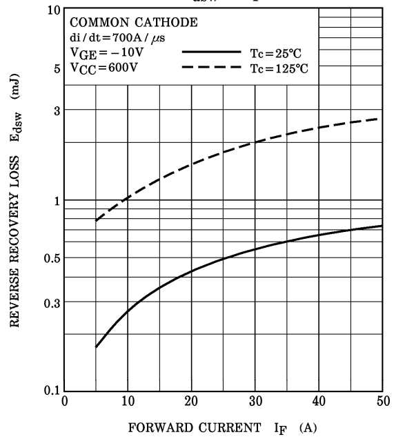
E_{dsw} - I_F
