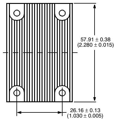
Figure 37. Longitudinal Heat Sink
