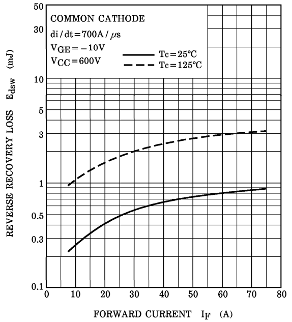
E_{dsw} - I_F
