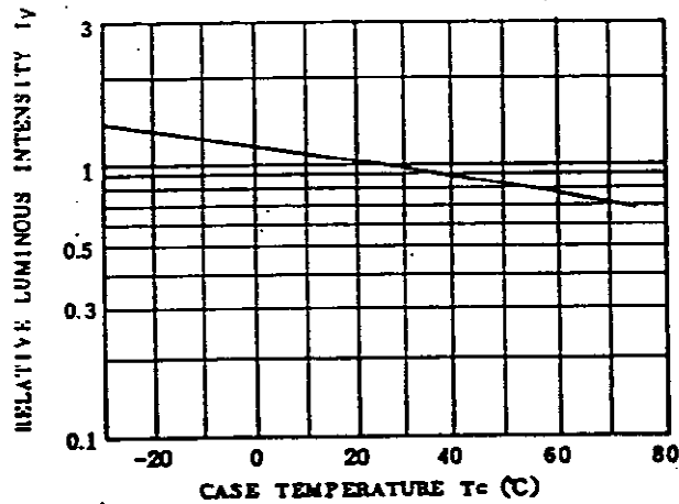
I_V - T_c
