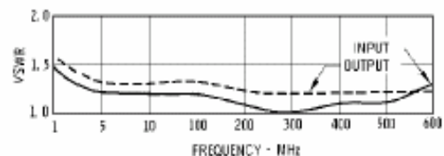
VSWR
