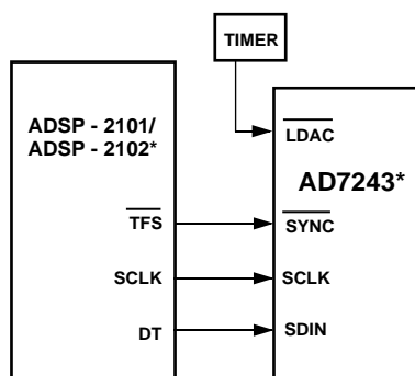
Figure 11. AD7243–ADSP-2101/ADSP-2102
