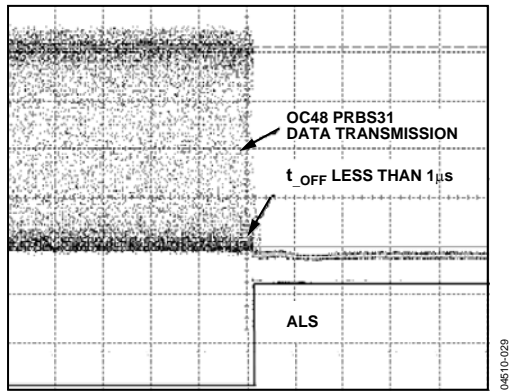
Figure 18. ALS Assert Time, 5 \mu\text{s/div}
