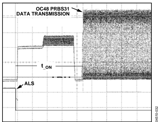
Figure 19. ALS Negate Time, 200 \mu\text{s/div}
