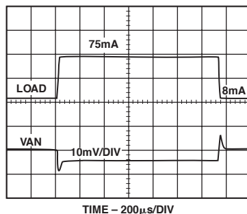
TPC 14. VAN Load Step
