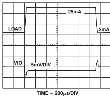
TPC 11. VIO Load Step
