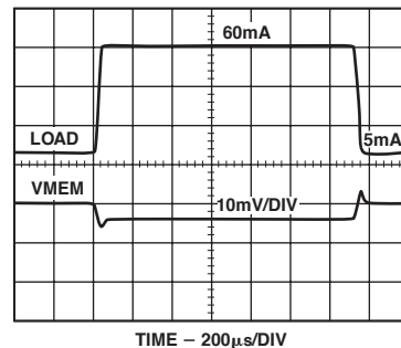
TPC 12. VMEM Load Step
