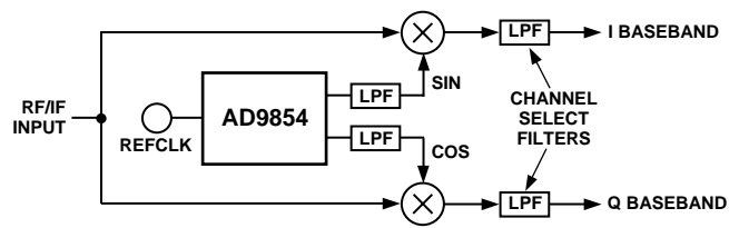
a. Quadrature Downconversion
