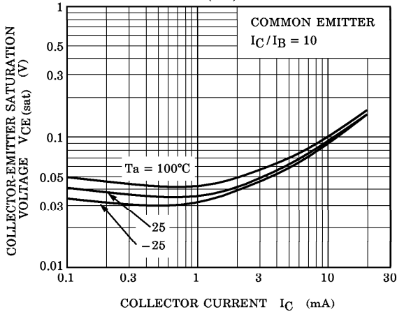
V_{CE(sat)} - I_C
