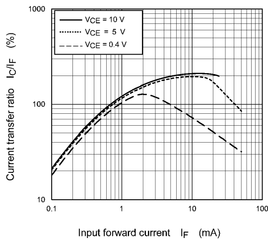
Fig. 11.10 I_C/I_F - I_F
