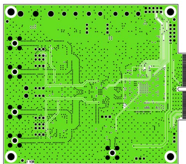
Figure 4. Layer 4, Bottom Layer
