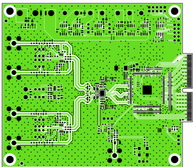
Figure 1. Layer 1, Top Layer
