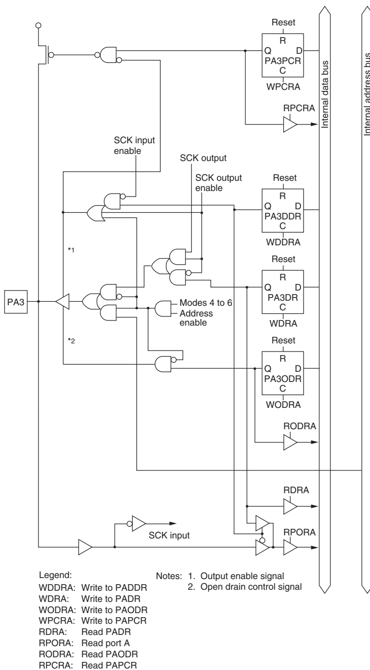
Figure C.6 (d) Port A Block Diagram (Pin PA3)
