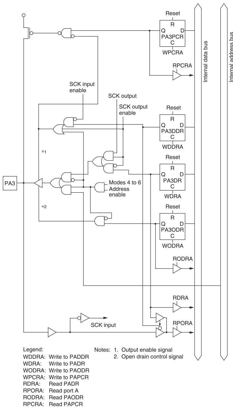
Figure C.18 (d) Port A Block Diagram (Pin PA3)
