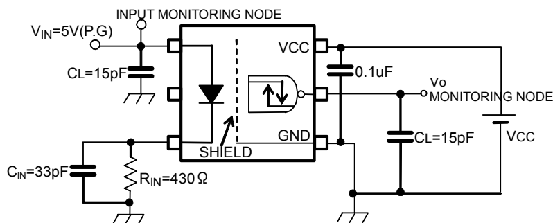
TEST CIRCUIT 2 : tpLH , tpHL
