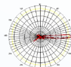
GD58-29 VPOL
